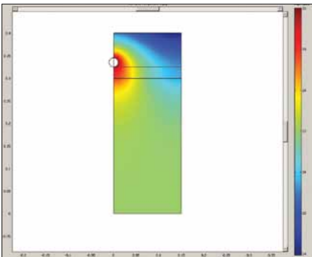
Billede 1: Finitiberegning af varmfordelingen i et betongulv
