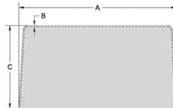
Maxi-Cover Aluminiumshætte VVS nr: 173951900
