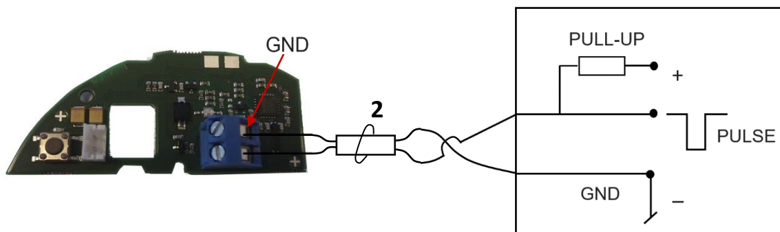
Skitse for tilslutning af pulsadapter
