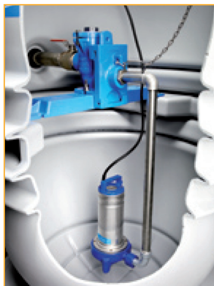
Dykket installation med hængende kobling til afgangsørret. Her i en Flygt Compit station.
