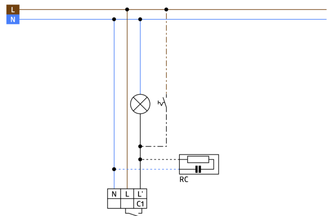
Ledningsdiagram
