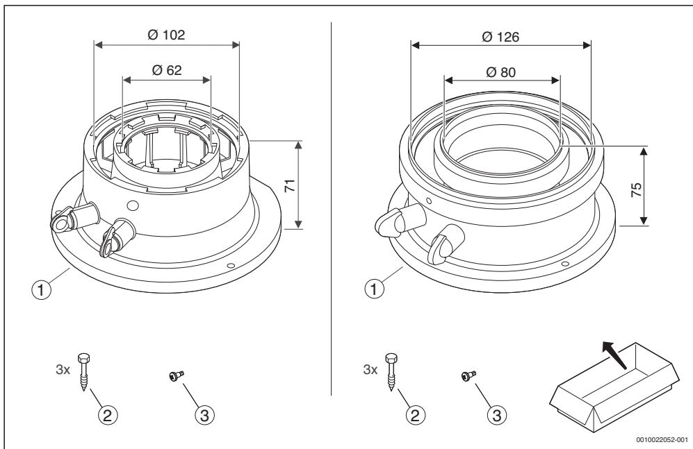
1 \text{Ø } 60/100 : 7738112636, \text{Ø } 80/125 : 7738112714
