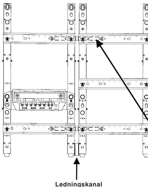
Sammenkoblingsbeslag, vandret Anbringes under DIN-skinner
