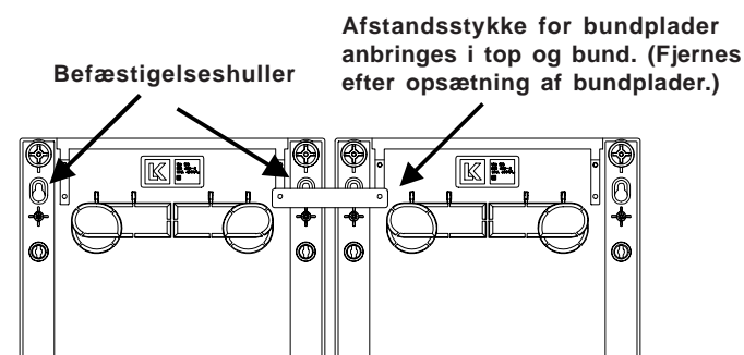
Sammenkoblingsbeslag, vandret
