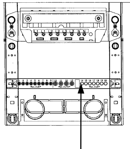
Afgreningsklemme
