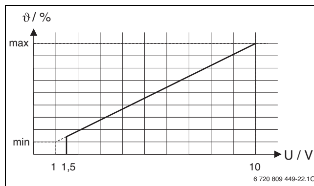
Fig. 2 Relazione lineare tra segnale da 0-10 V (tensione elettrica in Volt) e temperatura di mandata richiesta \theta (in percentuale riferita alla potenza massima dell'impianto)
