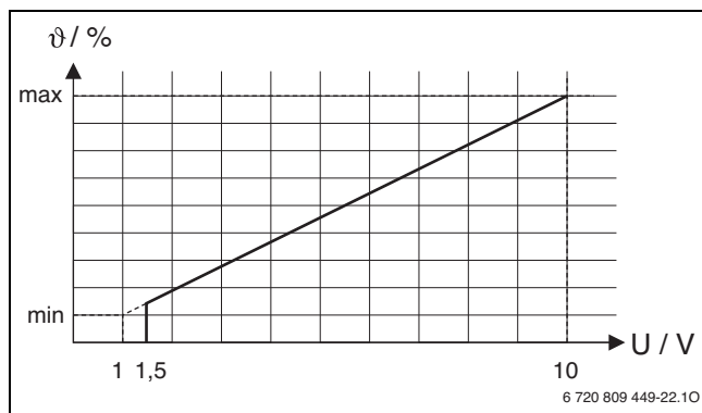
Bild 2 Linearer Zusammenhang zwischen 0-10 V-Signal ( U in Volt) und angeforderter Vorlauftemperatur \vartheta (in Prozent bezogen auf die Maximale Vorlauftemperatur)
