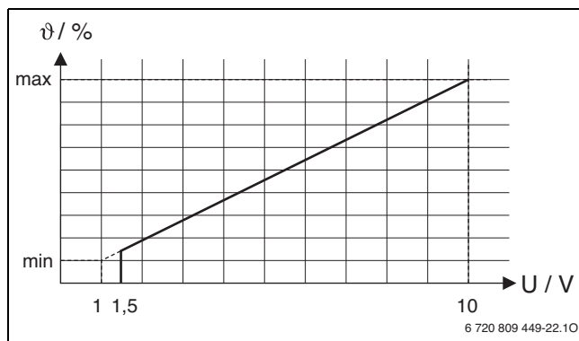
Fig. 2 Relation linéaire entre le signal 0-10 V ( U en Volt) et la température de départ \theta (en pourcentage par rapport à la température de départ maximale)
