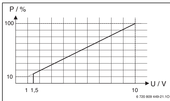
Fig. 1 Relación lineal entre la señal 0-10 V ( U en voltios) y la potencia P solicitada (en porcentaje en relación al rendimiento máximo del sistema)
