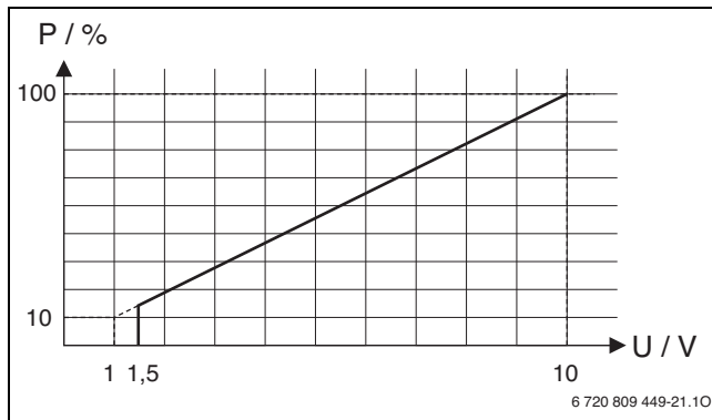
Afb. 1 Lineaire relatie tussen 0-10 V-signaal ( U in Volt) en gevraagde vermogen P (in procenten gerelateerd aan het maximale vermogen van de installatie)
