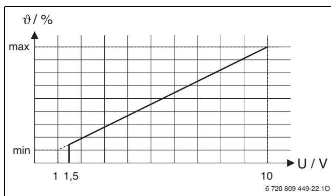
Fig. 2 Relación lineal entre señal 0-10 V ( U en voltios) y temperatura de impulsión solicitada \theta (en porcentaje, en relación a la máxima temperatura de impulsión)
