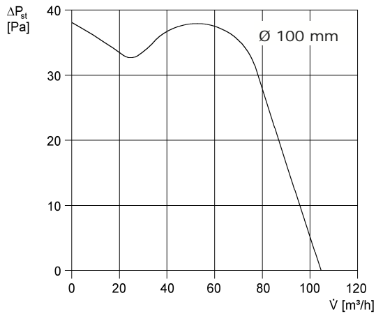
Modtryksdiagram
